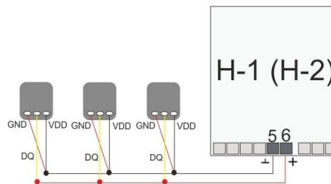
Датчик DS18B20
