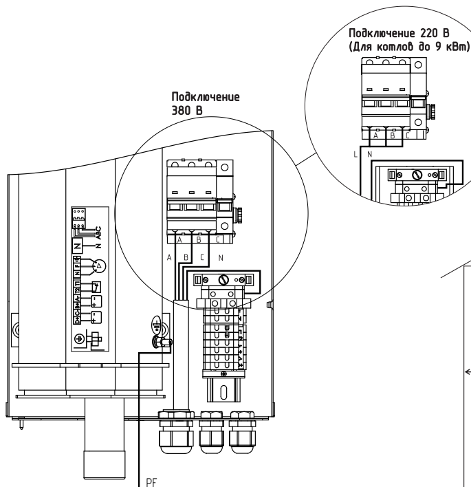
Рис. 3 Схема подключения электроводонагревателя
