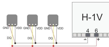
Датчик DS18B20
